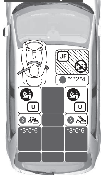
Airbag passager activé pour modèle à conduite à gauche
